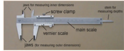
القدمة ذات الورنية
