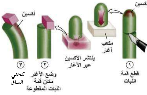
الشكل (٢٤): تجارب العالم فنت لاكتشاف دور الأكسين.
